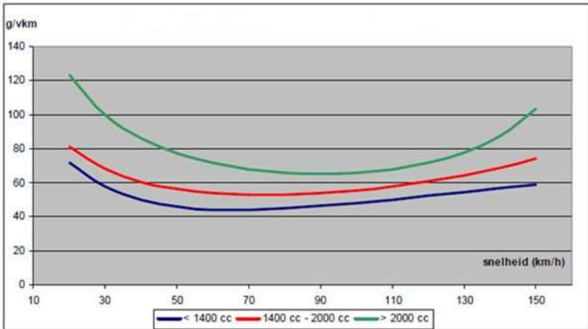
Figuur 14: Brandstofverbruik van benzine wagens (per cc-klasse)
